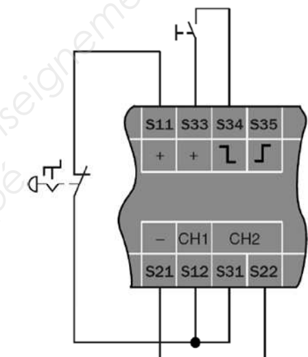
Schéma ARU et réarmement manuel
