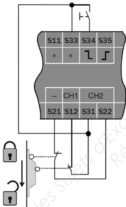
Schéma protection porte et réarmement manuel
